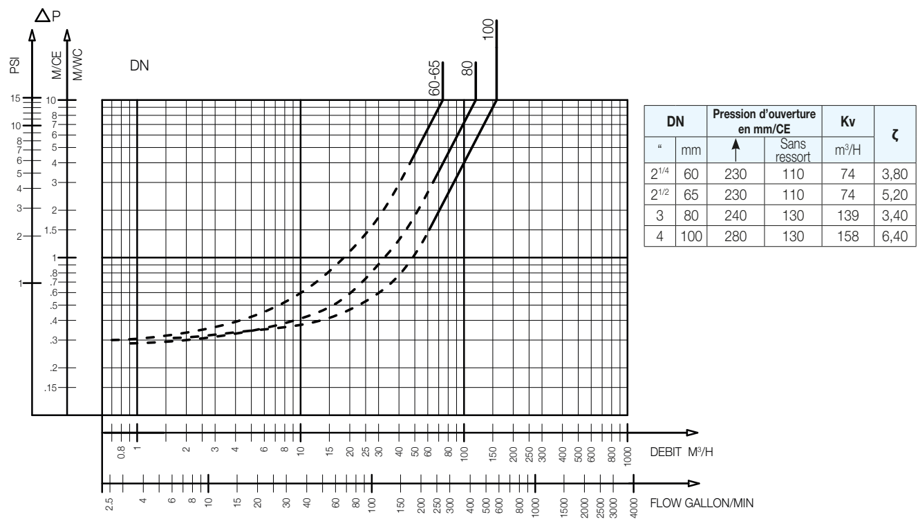
102 - Abaque des pertes de charge
